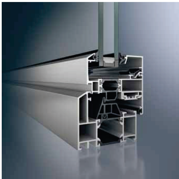
Schüco Raam AWS 65 RL Systeem met afgeschuinde buitenlijst Fenêtre Schüco AWS 65 RL Système avec cadre extérieur biseauté
